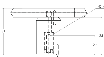
T Knob
